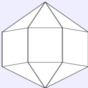
方解石
