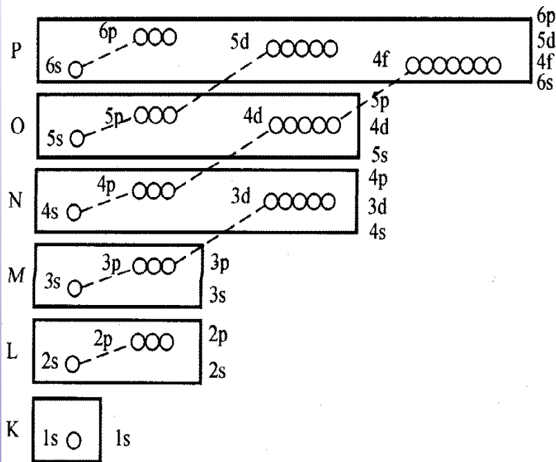
多电子原子的近似能级图
