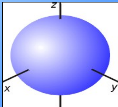
s 轨道 球形
