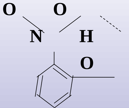
邻硝基苯酚
