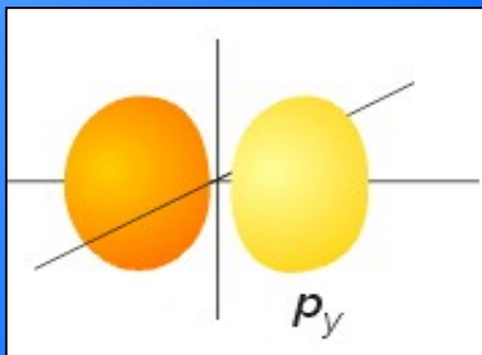
p 轨道 哑铃形 双纺锤体
