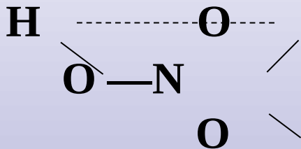
硝酸
