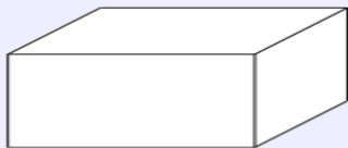
食盐
